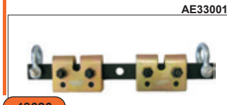
Зажим для кузовных работ, 2 направления, усилие 5 т AE330015
