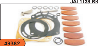
Ремонтный комплект для пневматического гайковерта JAI-1138 JAI-1138-RK
