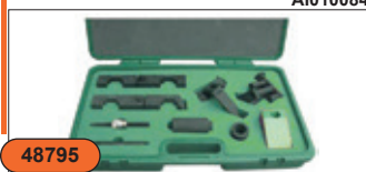
Набор для регулировки ГРМ VANOS двигателей BMW V8 M60/M62/M54 AI010084
